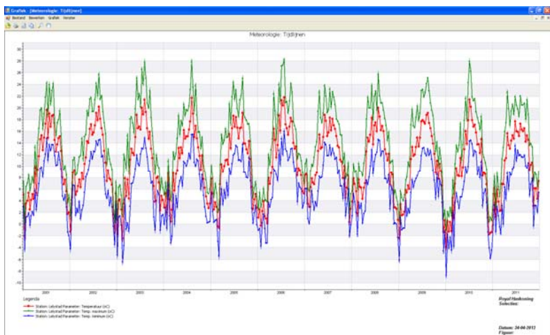
Figuur 14: Temperatuur gegevens station Lelystad
