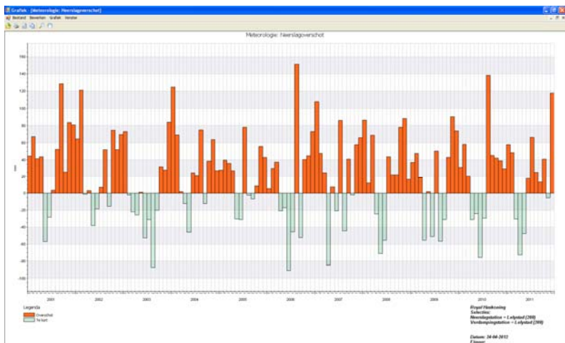
Figuur 13: Neerslagoverschot station Lelystad
